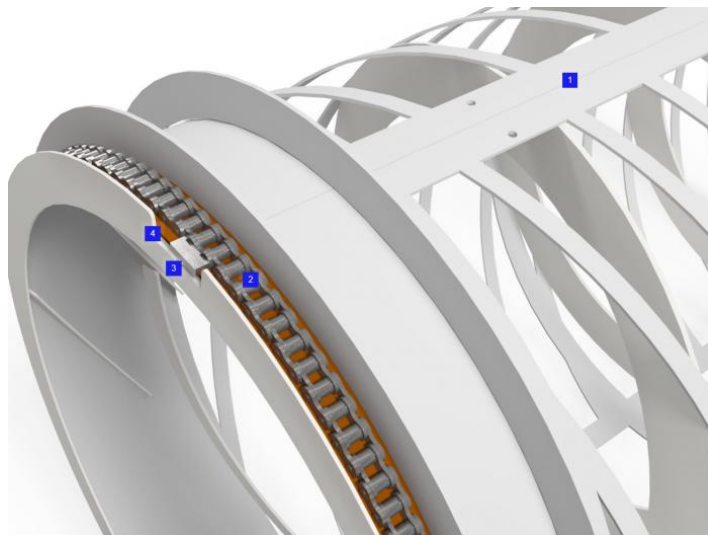
(Abb. Kettenschloss)
